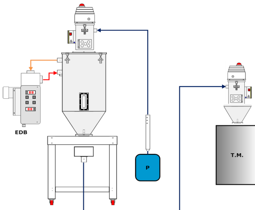
EDB – Instalación sobre bancada/carrito.
