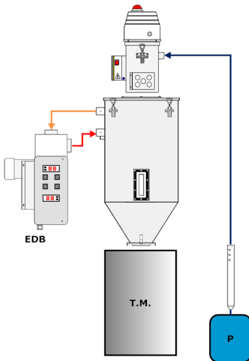
EDB – Instalación sobre una maquina transformadora
